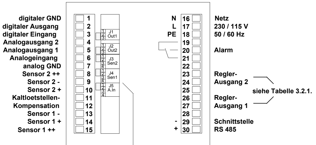
Codier - Jumper für Sensoren und analoge Ein bzw. Ausgänge
